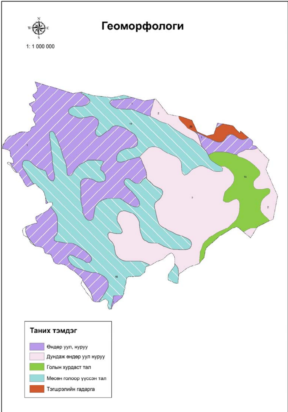
Зураг №36. Геоморфологи
