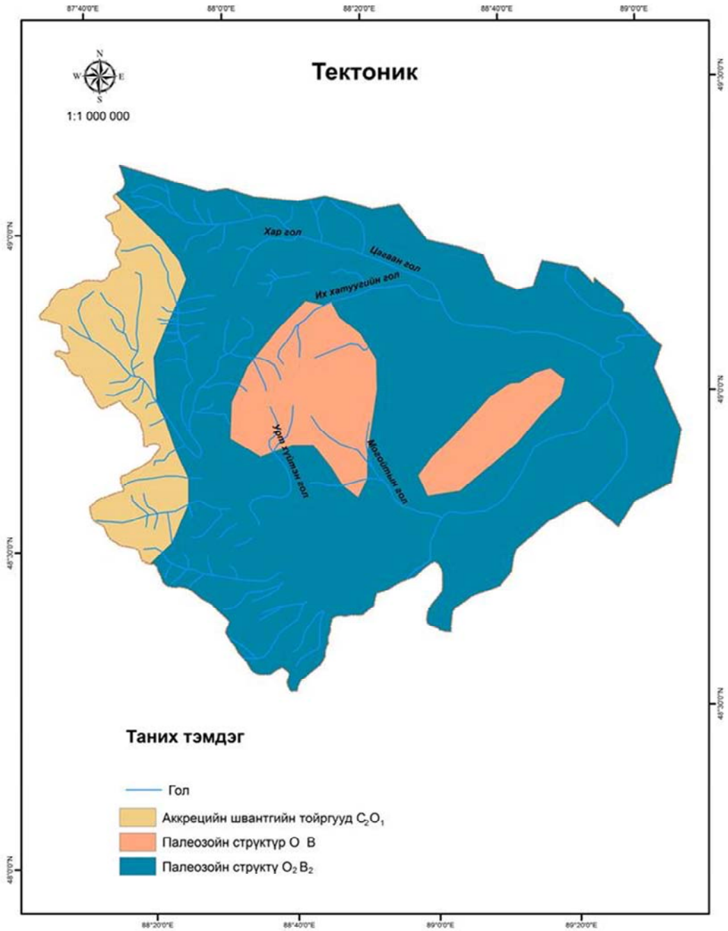
Зураг 38. Тектоник
